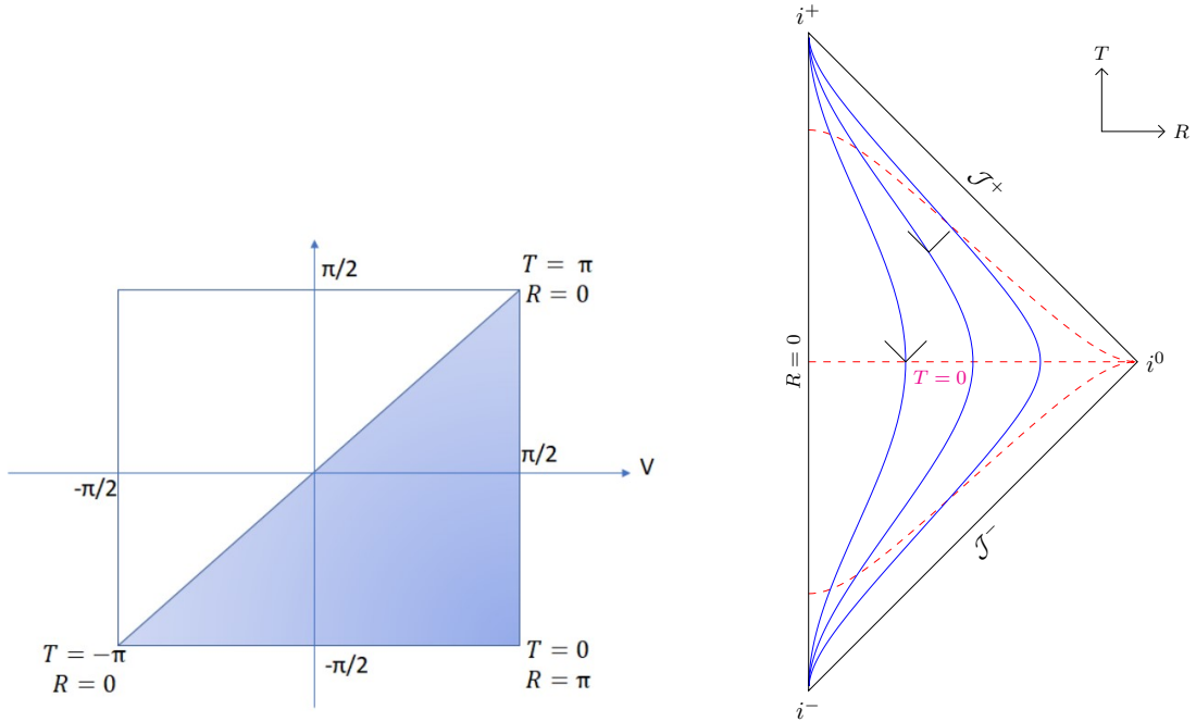
(a) Espace (conformellement) de Minkowski (bleu) dans les coordonnées (U, V) . Note : les coordonnées (T, R) sont ici changés d'un facteur 2.
