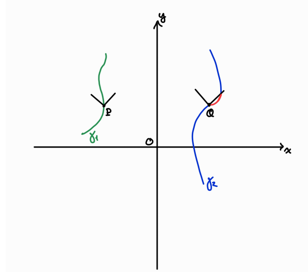
FIGURE 2.3 – En \mathbb{R}^{1,3} , uniquement les trajectoires du type \gamma_1 sont admissibles. La courbe \gamma_2 ne peut pas représenter la trajectoire d'une particule car son tracé n'est plus contenu dans le cône de lumière de Q .
