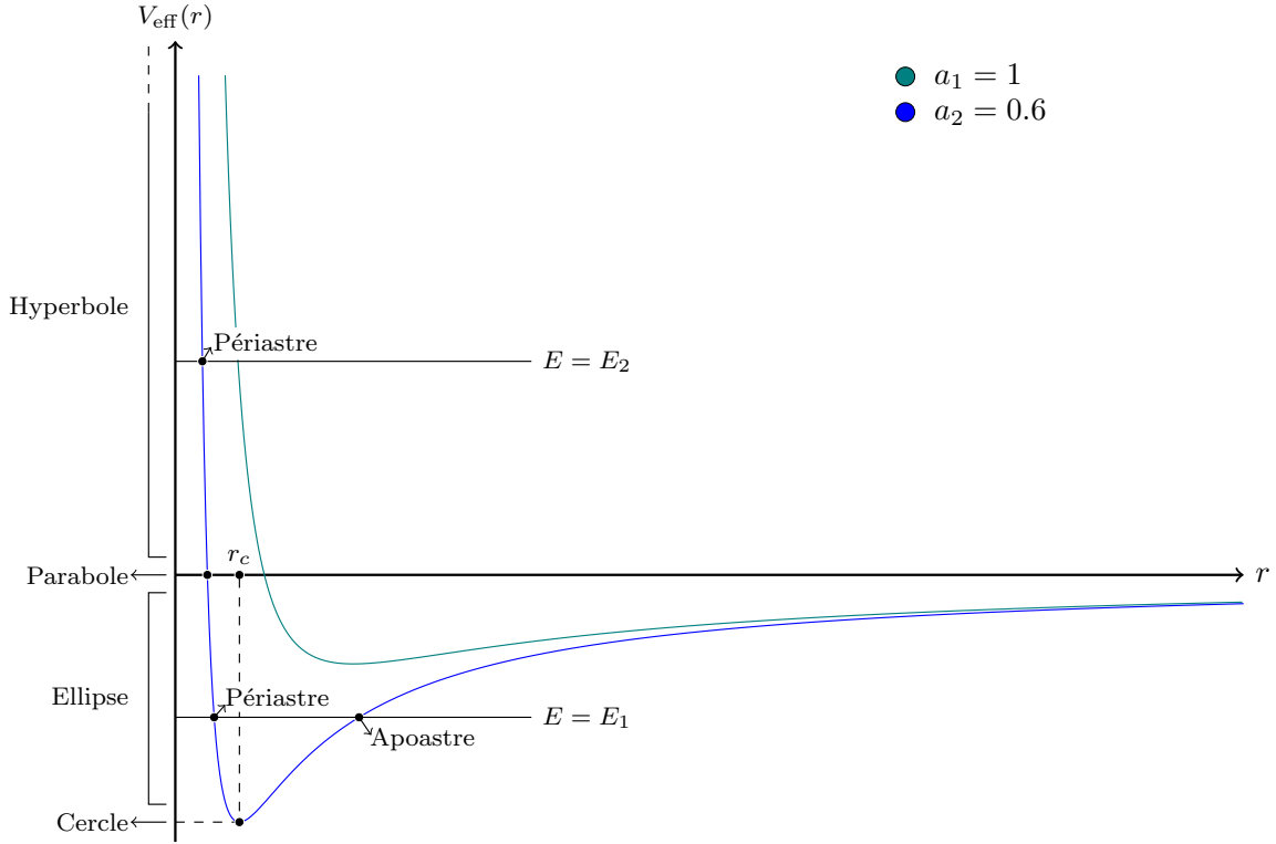
FIGURE 7.1 – Représentation du potentiel pour deux valeurs de a (et GM = 1 ). Différentes valeurs d'énergie des particules vont déterminer le type de mouvement suivi. Deux énergies y sont illustrées, pour lesquelles la particule suit soit une ellipse ( E_1 ) ou une hyperbole ( E_2 ).
