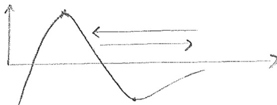
FIGURE 7.2 – Illustration d'une orbite non-bornée.
